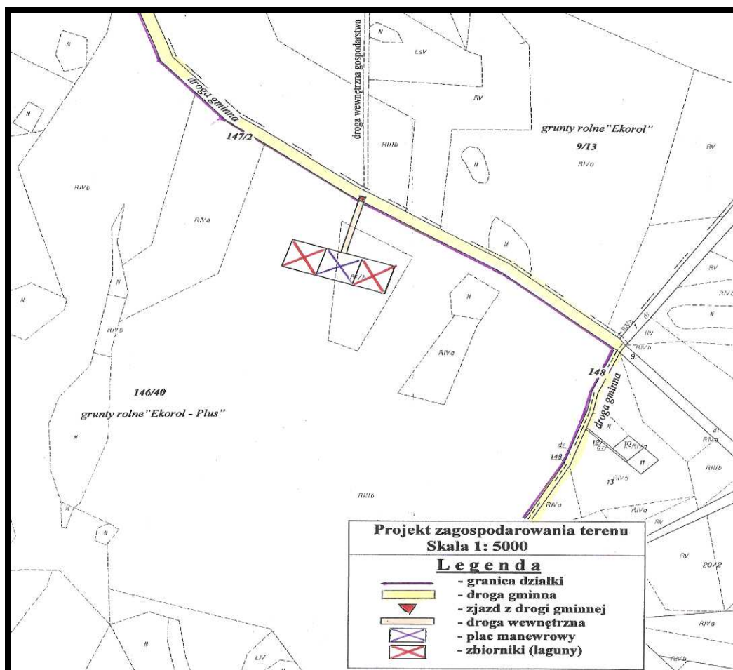
Ryc. 3. Projekt zagospodarowania terenu inwestycji
