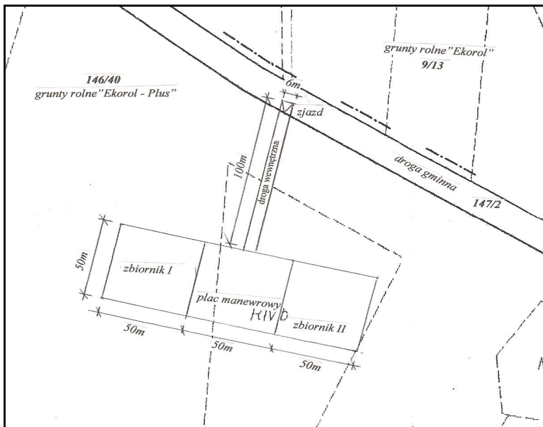
Ryc. 2. Wymiary projektowanych obiektów budowlanych
