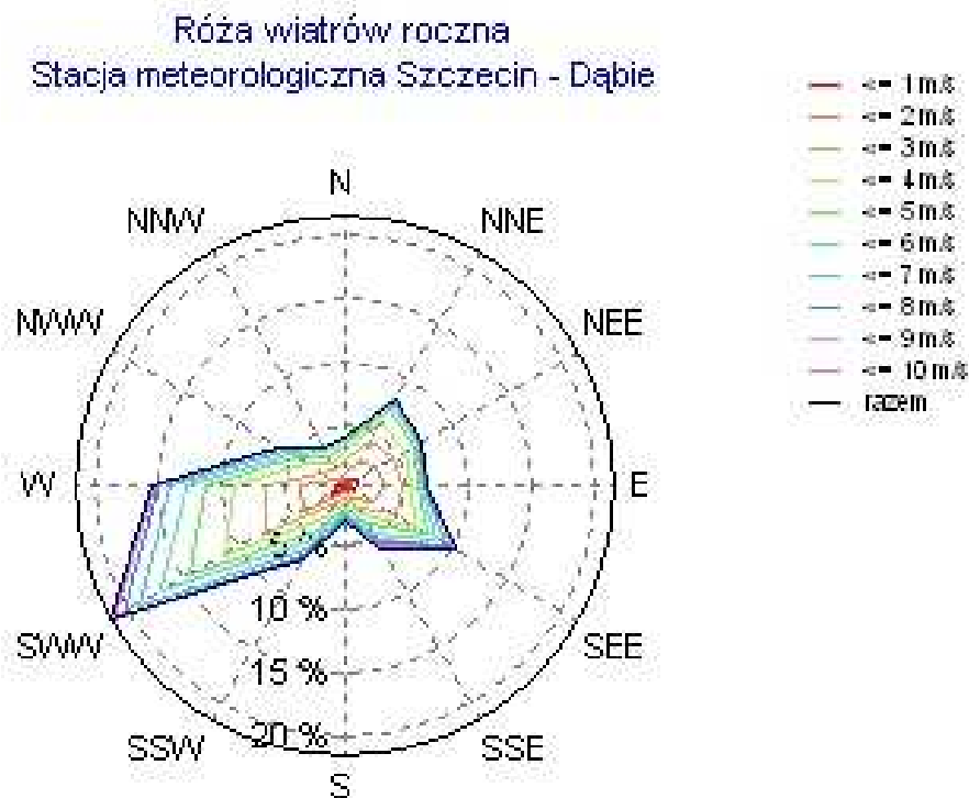
Ryc. 38. Roczna róża wiatrów dla stacji meteorologicznej nr 205 Szczecin Dąbie (interpretacja graficzna)
