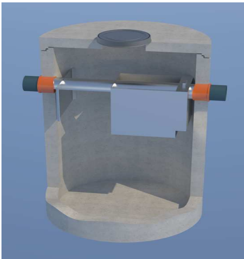
Ryc. 36. Rysunek separatora- przekrój
